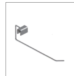
일공행거 A: 130mm B: 180mm C: 230mm D: 280mm
