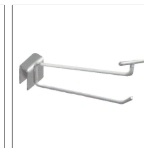
2단 가격표지 후크 A: 100mm B: 150mm C: 200mm D: 250mm E: 300mm
